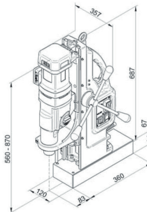
MAB 1300 V
