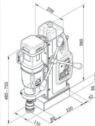
MAB 845
