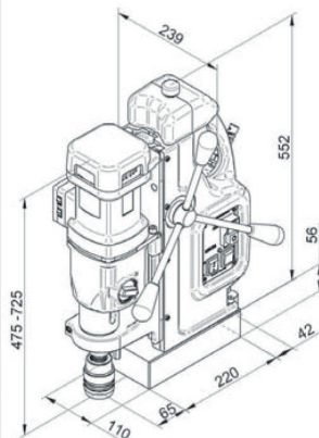
MAB 845
