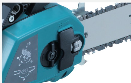
Udskiftning af kæde og kædebespænding uden brug af værktøj (EA3501S, EA3201S)
